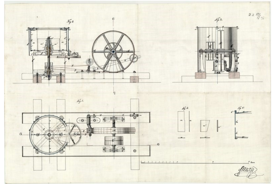
Patenttegningen af mælkecentrifugen fra Maglekilde Maskinfabrik. 1878. Rigsarkivet
